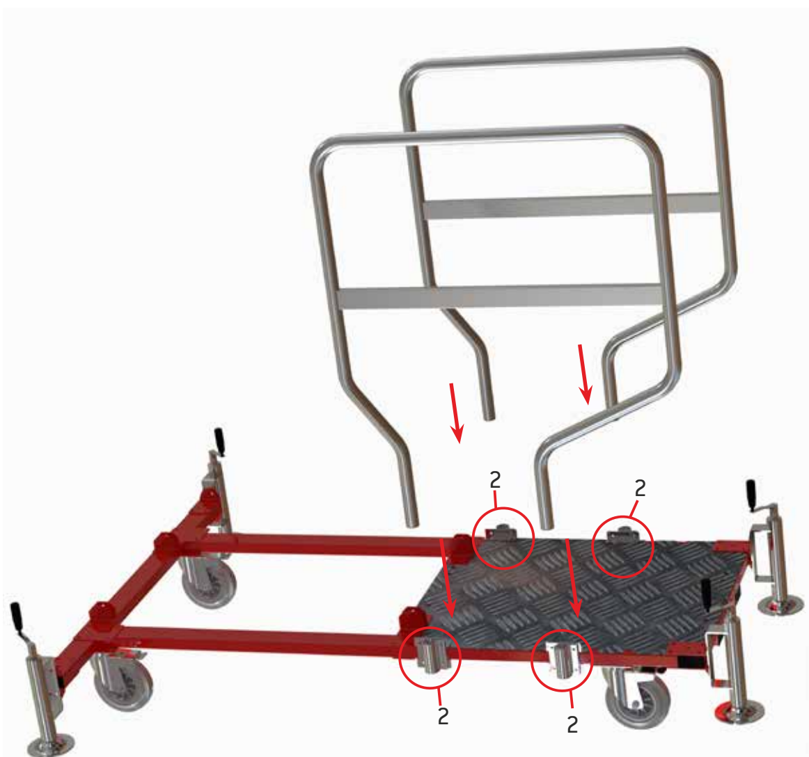
DETALLE 2
