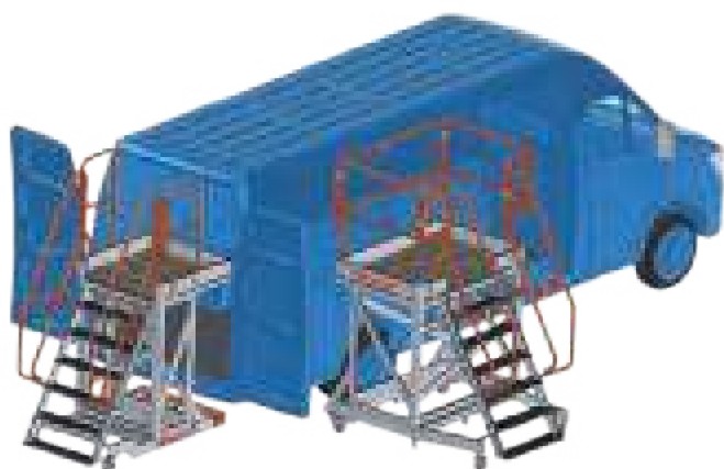
EM111 Estructura a Medida Estrutura à medida
