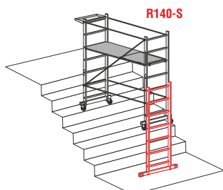
Kit escalinatas. Kit escadarias.
